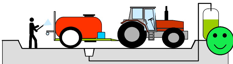
Fig. 96 - Area attrezzata per il lavaggio dell'irroratrice e per il convogliamento delle acque di lavaggio in appositi serbatoi di raccolta.
