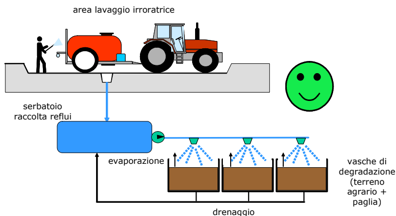
Fig. 95 - Raccolta delle acque reflue del lavaggio e loro biodegradazione (biobac ®). Il contenuto delle vasche di degradazione viene monitorato e periodicamente arieggiato e rovesciato e deve essere sostituito ogni circa 5 anni. Tale terreno esausto può poi essere distribuito in campo
