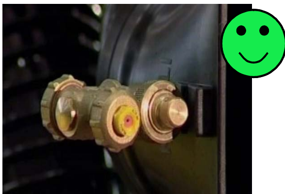
Fig. 36 – Particolare di ugello abbinato ad antigoccia.
