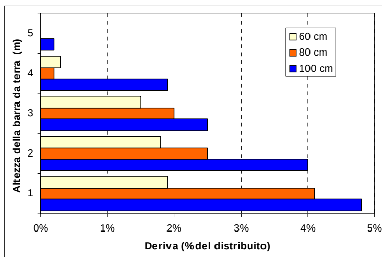
Fig. 53 – E' sempre opportuno mantenere l'altezza da terra della barra la più bassa possibili per ridurre la possibilità di deriva del prodotto fitoiatrico.
