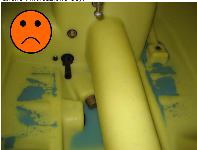
Fig. 39 – Miscela residua nel serbatoio poiché non aspirata dalla pompa (foto E. Nilsson – Visavi)
