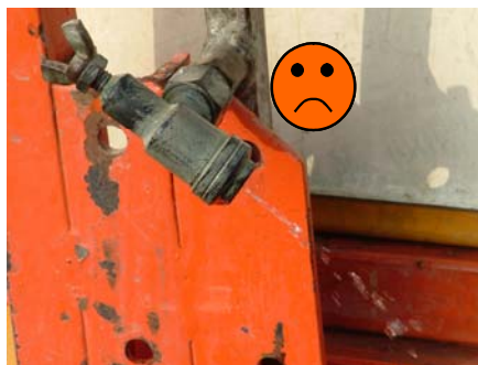
Fig. 37 - Esempio di ugello NON dotato di dispositivi antigoccia (sinistra) e di antigoccia non funzionante (destra).
