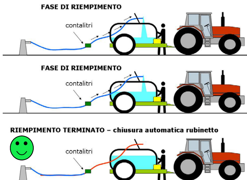
Fig. 54 – Quando sul contalitri si è raggiunto il volume preimpostato, automaticamente tramite la chiusura di un rubinetto si interrompe l'invio dell'acqua nel serbatoio principale.
