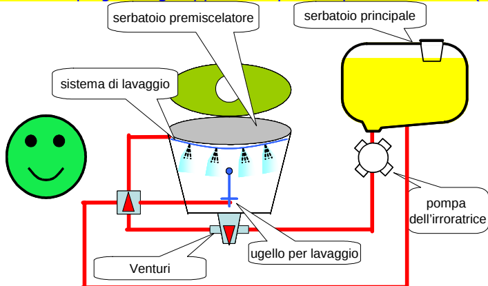
Fig. 65 – Il serbatoio premiscelatore consente l'aspirazione dei formulati, il corretto dosaggio, la premiscelazione del prodotto, l'introduzione del prodotto nel serbatoio principale, il lavaggio dei contenitori vuoti di agrofarmaci.
