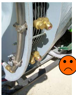
Fig. 37 - Esempio di ugello NON dotato di dispositivi antigoccia (sinistra) e di antigoccia non funzionante (destra).
